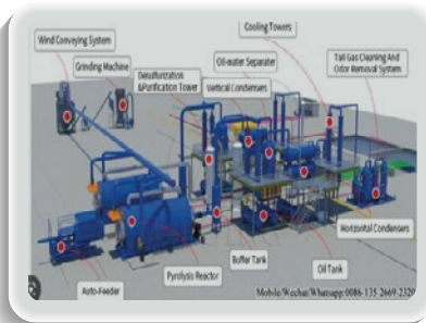
Quá trình nhiệt phân
